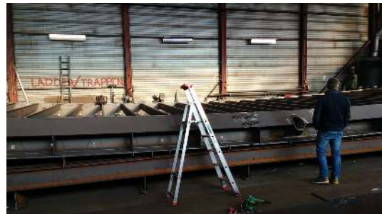
Afbeelding 8. Brugdek (2)
